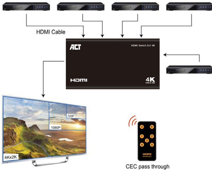
Anschlusschema 1 (Unterstützung 4Kx2K)
