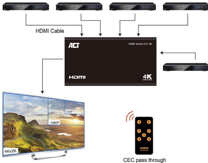
Tilkoblingsdiagram 1 (støtte 4Kx2K)
