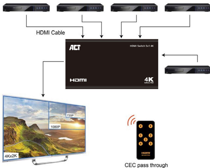
Diagrama de conexión 1 (Soporta 4Kx2K)
