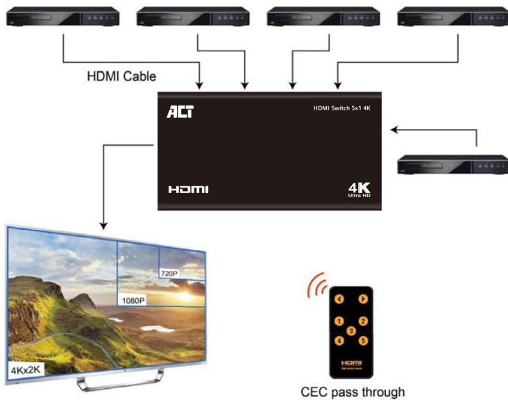
Tilslutningsdiagram 1 (understøtter 4Kx2K)
