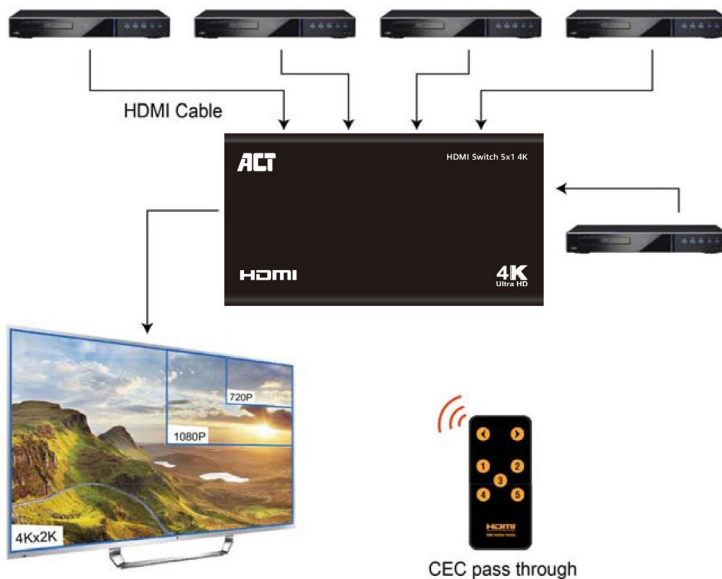
Liitäntäkaavio 1 (tuki 4Kx2K)
